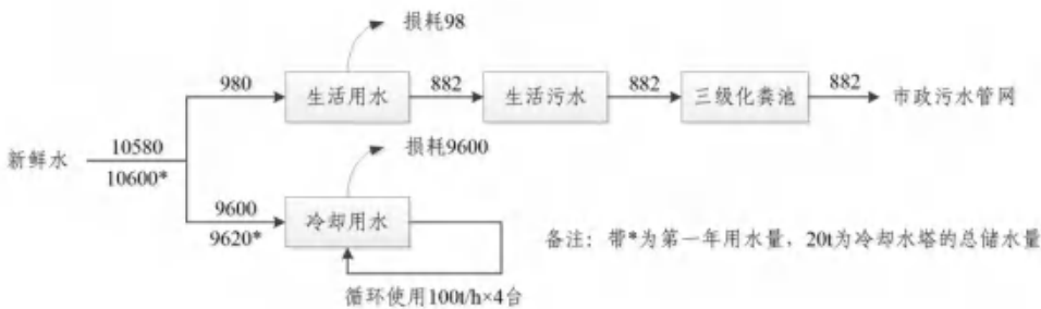
图 2-2 本项目水平衡图 单位：t/a
