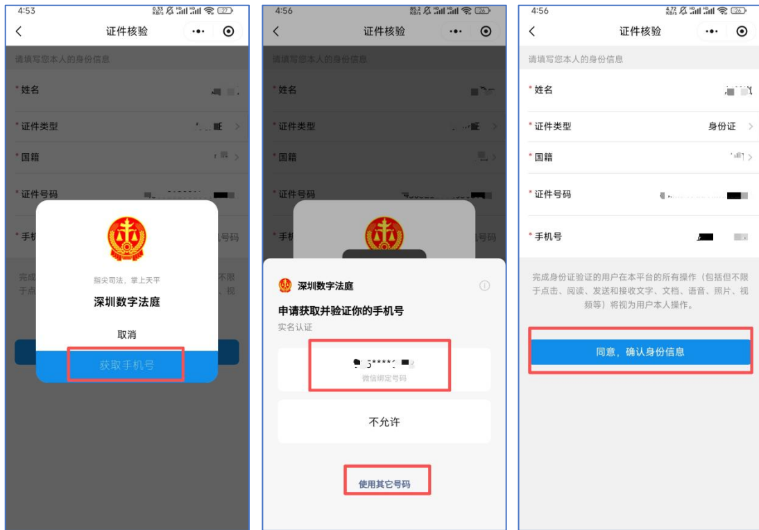
图 1.1-3 获取手机号
