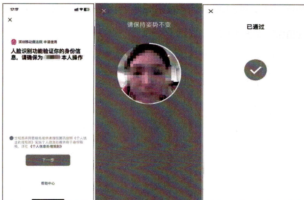
图 1.1-4 人脸识别
