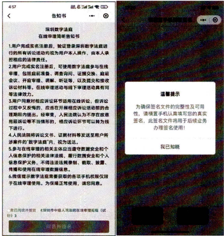
图 1.1-5 在线签名
