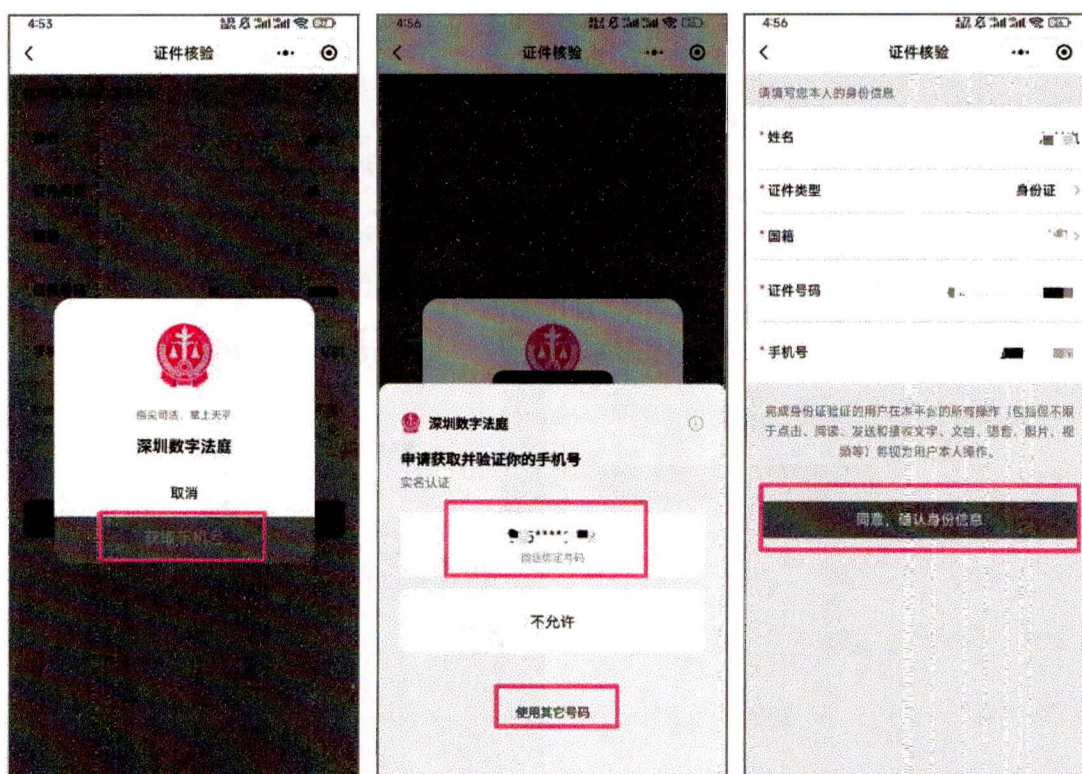
图 1.1-3 获取手机号
